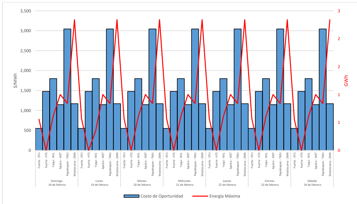
Figura 8b. Costos de Oportunidad y Energía Hidro Máxima Diaria por Embalse en el MDA.
