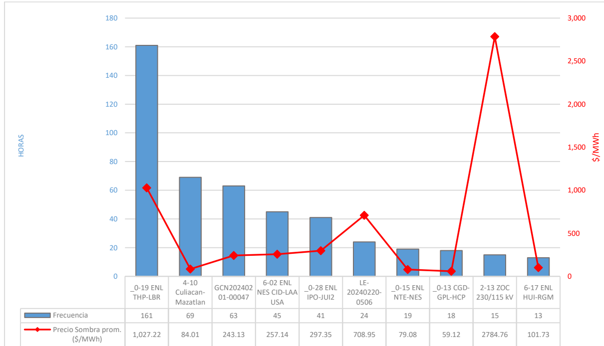
Figura 9a. Frecuencia de Enlaces de Transmisión Congestionados en el MDA.
