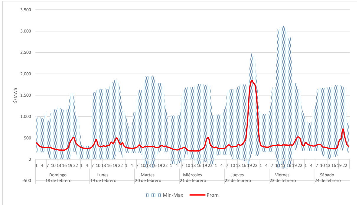
Figura 5. Precio Marginal Local Promedio en el MDA.
