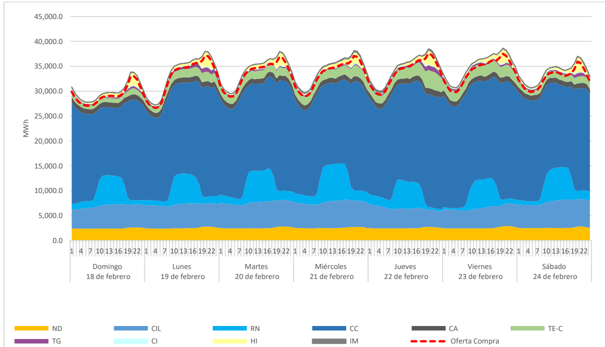
Figura 3. Oferta total de compra y despacho con desglose de la Oferta Térmica en el MDA.
