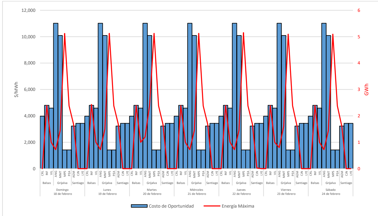
Figura 8a. Costos de Oportunidad y Energía Hidro Máxima Diaria por Embalse en el MDA.
