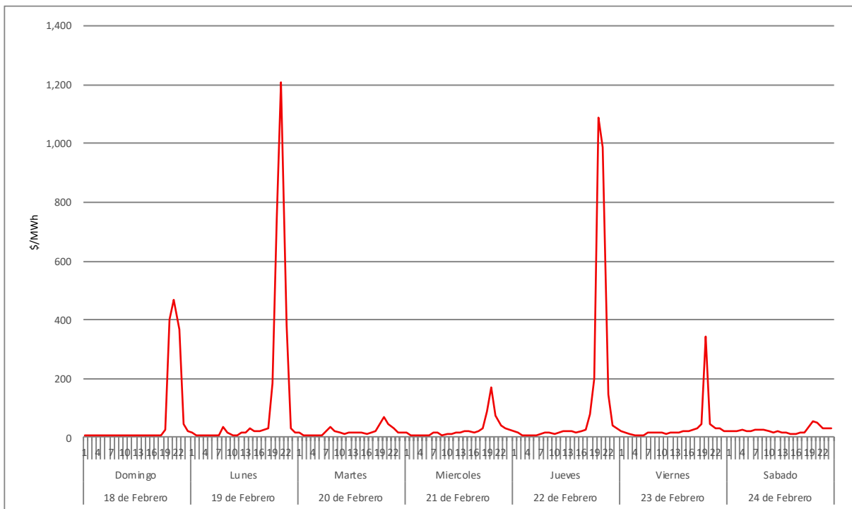
Figura 17. Precio de la Reserva Rodante de 10 minutos.
