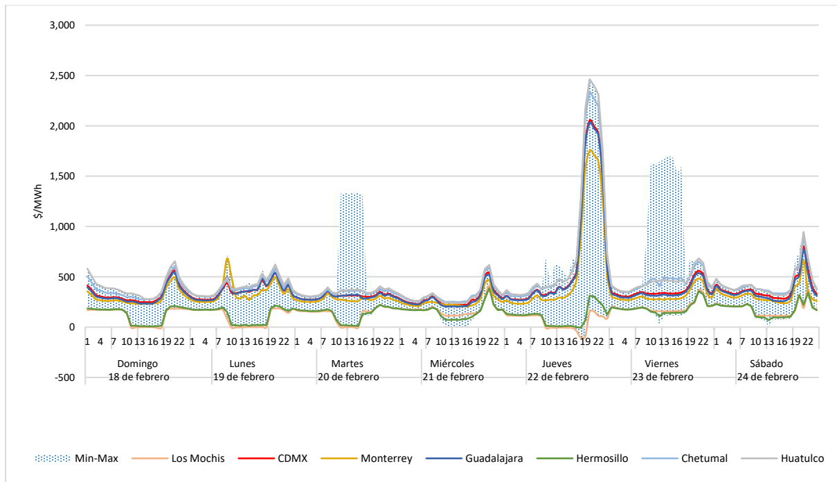
Figura 6. Precios en Nodos Distribuidos (Zonas de Carga) Representativos en el MDA.
