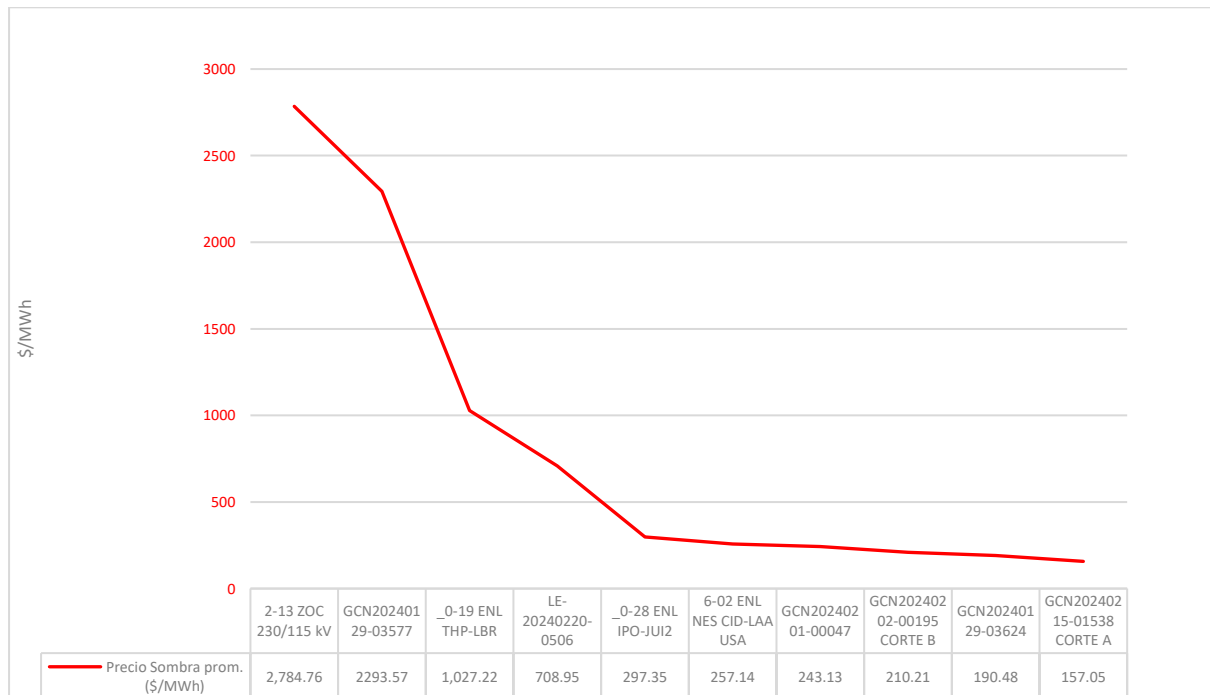
Figura 9b. Precio Sombra promedio de Enlaces de Transmisión Congestionados en el MDA.
