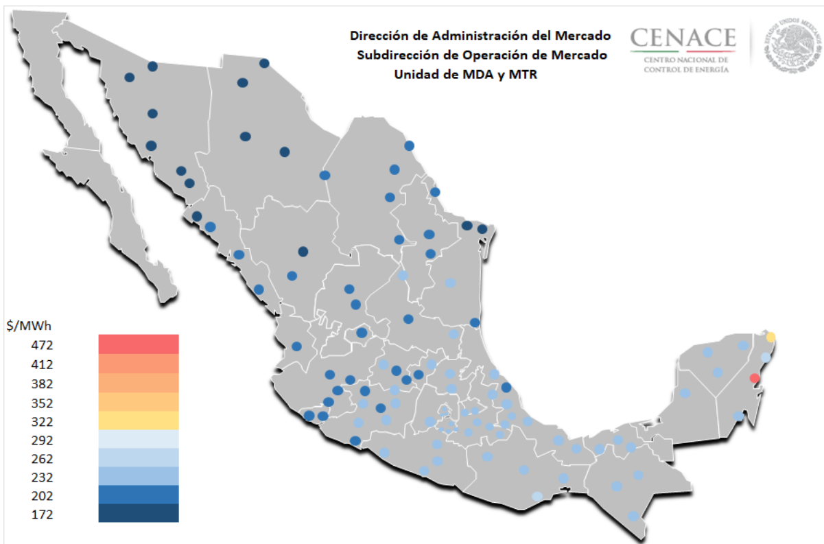
Figura 15. Precio Promedio Semanal en Nodos Distribuidos (Zonas de Carga) en el MTR ex-post.
